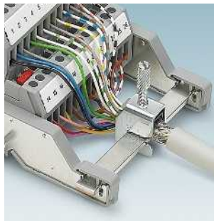
Экранированные опоры для нейтральных магистральных шин AB-SK ..., AB/SS ... Стр. 576
