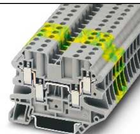
39 А, проходные и заземляющая клемма, 4 разъема
