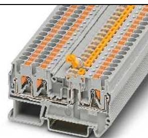
20 А, клемма с ножевым размыкателем, 3 разъема
