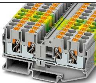
52 А, проходной блок зажимов, 4 разъема
