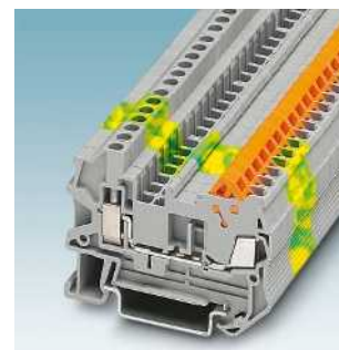
Гибридные клеммы с односторонним винтовым разъемом 1,5 мм² ... 2,5 мм² ...
