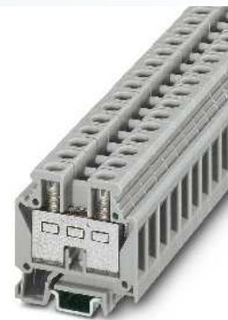
6 (10) мм 2 , 57 А, проходная клемма
