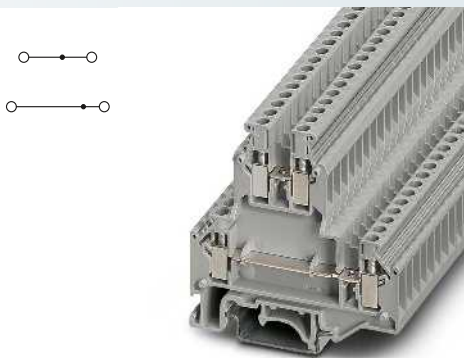
4 (4) мм², 32 А, двухъярусная клемма, возможность установления перемычки на обеих ярусах
