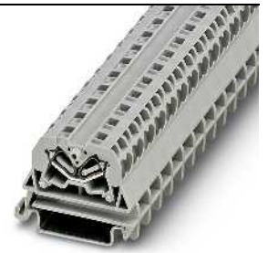
30 А, проходной блок зажимов, боковой кабельный ввод, 4 разъема
