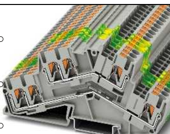
24 А, двухъярусная клемма, 3 разъема на ярус
