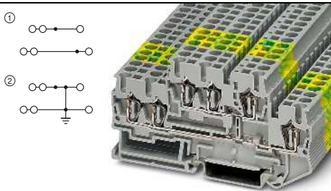
26 А, проходной блок зажимов, 3 разъема на каждом ярусе
