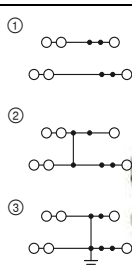
24 А, двухъярусная клемма, 3 разъема на ярус
