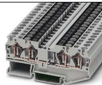
37 А, проходной блок зажимов, 4 разъема, с обесточенной сборной шиной
