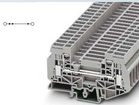
6 (10) мм 2 , 57 А, проходная клемма, с одина- ковыми контурами
