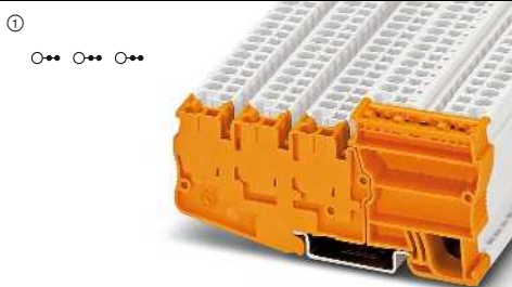
30 А, клеммный модуль питания
