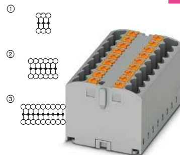
24 А, прилеивание
