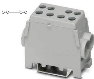
25 (35) мм 2 , 125 А, отводная клемма для основной линии, 2 отвода по 25 мм 2
