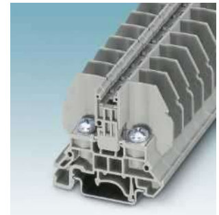
Болтовые клеммы для установки на монтажную рейку и прямого монтажа RSC ...
