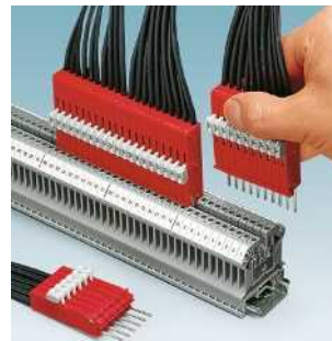
Тестовый штекер для клемм серии UK MPS ... PS-UK ...
