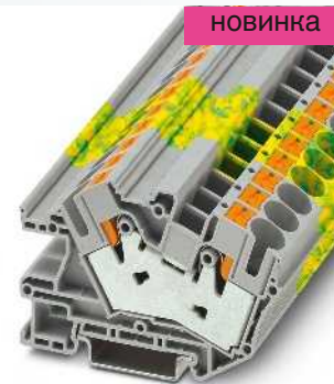
76 А, проходной блок зажимов
