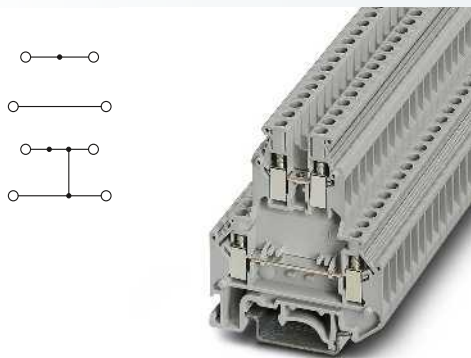
4 (4) мм², 32 А, двухъярусная клемма
