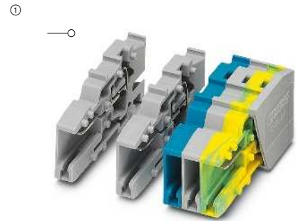
24 А, устройство сопряжения, самостоятельная сборка
