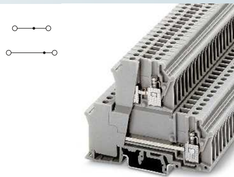
4 (4) мм², 32 А, 800 В, двухъярусная клемма, возможность соединения обоих ярусов перемычкой
