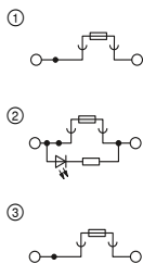
10 А, клемма с держателем предохранителя (для стеклянных предопр.) 5 x 20 мм
