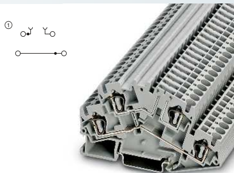
34 А, двухъярусная клемма разделительной зоной
