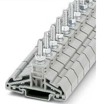
35 (35) мм 2 , 125 А, М6 болтовая клемма
