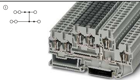
26 А, проходной блок зажимов, с объединением потенциалов
