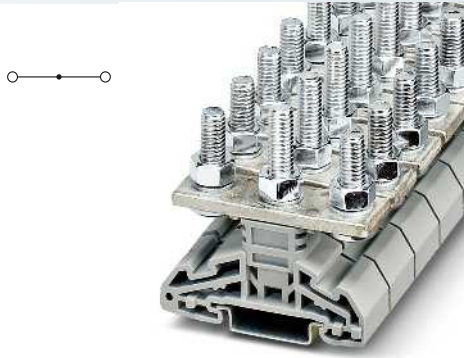
50 (50) мм 2 , 150 А, М8 болтовая клемма
