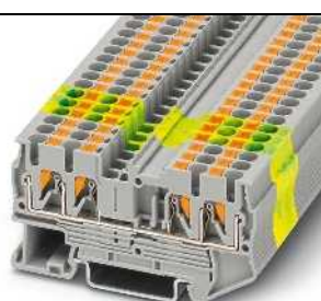
28 А, проходная клемма, 4 разъема
