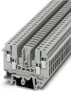
4 (6) мм 2 , 16 А, разделительная клемма
