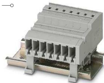
32 A, устройство сопряжения для монтажа на несущей рейке
