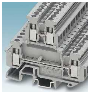
Двухъярусные миниатюрные клеммы МВККВ ... Стр. 530
