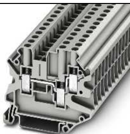
39 А, 1000 В, проходная клемма, 3 разъема
