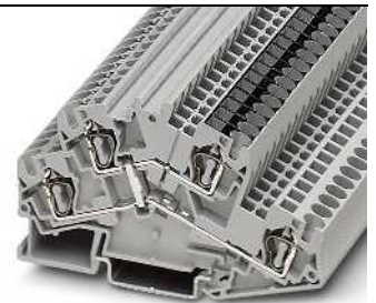
34 А, двухъярусные клеммы, с объединением потенциалов
