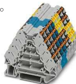
20 А, распределитель потенциалов, 16 разъемов
