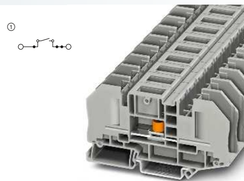
41 А, разделит. клемма для измерит. преобразователя, открытая
