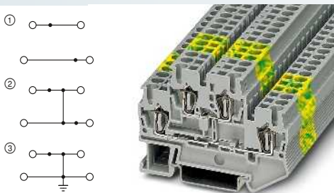
26 А, двухъярусные клеммы
