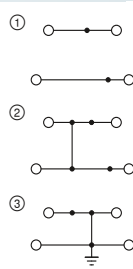
36 А, двухъярусная клемма
